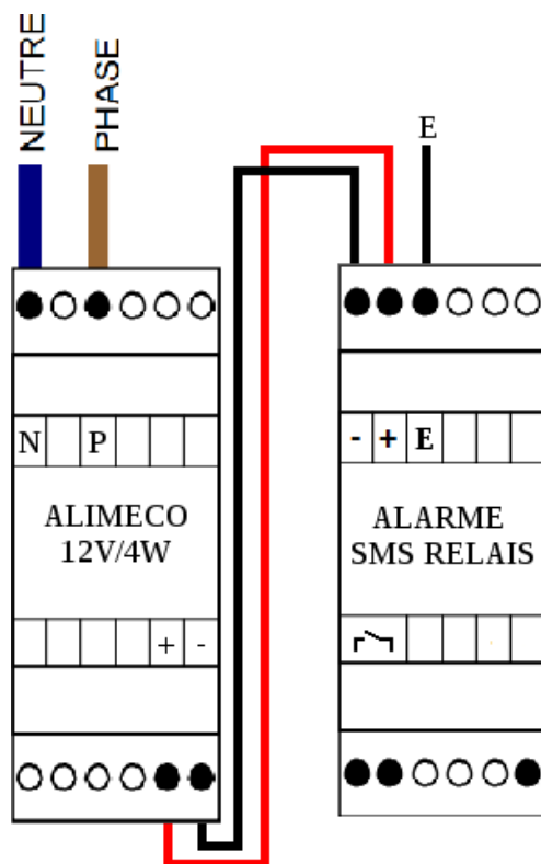
Réf. 1263 : alimentation 12V DC
